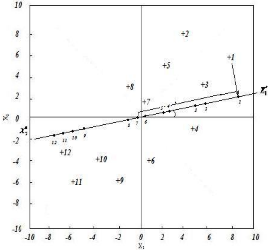
Şekil 3.2. Ortalamaya Göre Düzeltilmiş Birimlerin Değerlerinin X_1^* Eksen Üzerindeki İz Düşümleri
