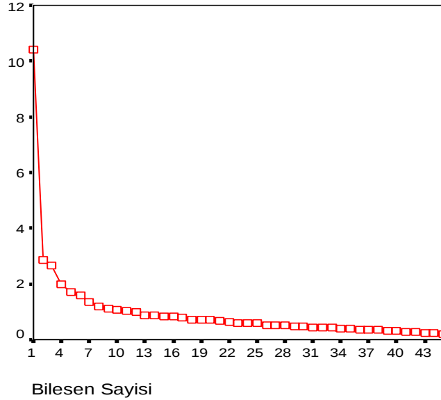
Şekil 4.1. Özdeğerler Grafiği (Scree Plot)
